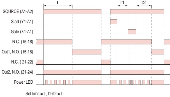
输出模式B:闪烁(OFF先计时)
