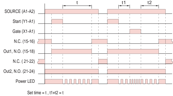
输出模式D1:信号OFF计时(信号OFF输出)
