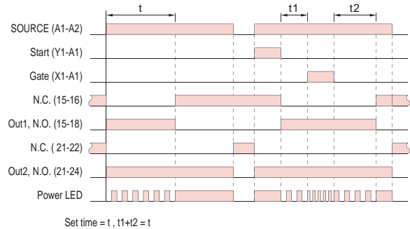
输出模式E1:反动作(信号OFF计时)
