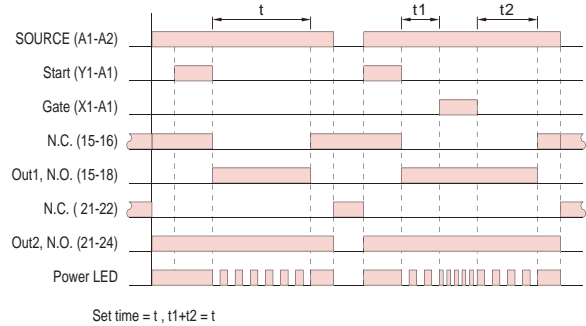
输出模式E:反动作(信号ON计时)
