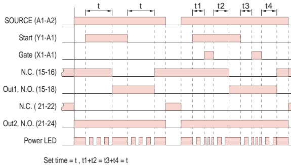
输出模式C:信号ON-OFF计时
